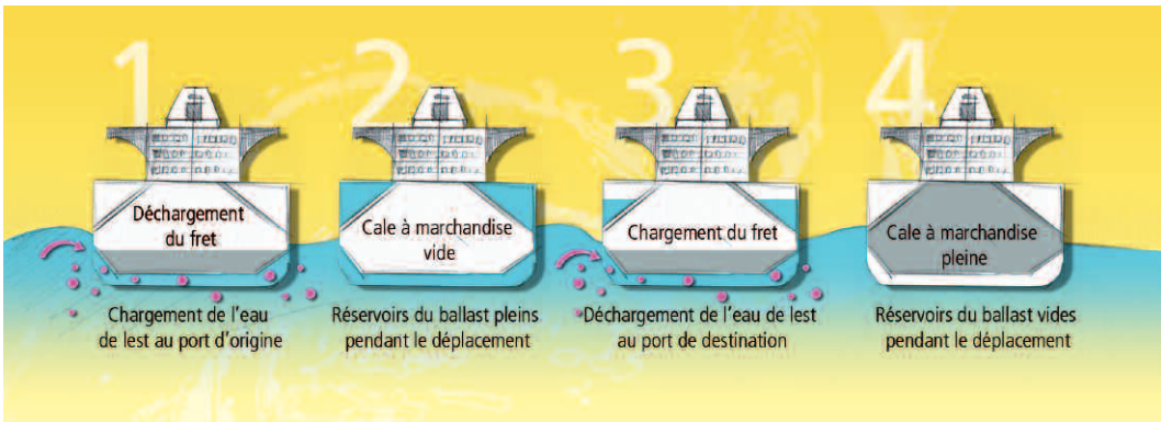
Vue transversale d'un navire montrant les réservoirs de ballast et le cycle suivi par l'eau de lest. Adapté du Fonds mondial privé pour l'environnement, Programme des Nations Unies pour l'environnement, Organisation maritime internationale, Programme mondial de gestion de l'eau de lest (programme GloBallast), 2007.
