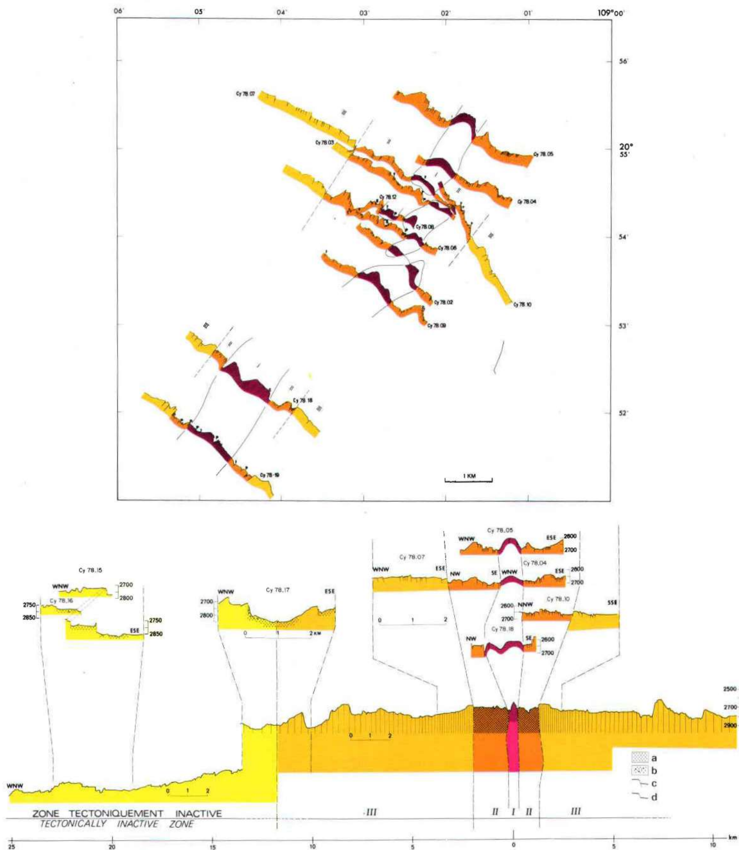
Coupes synthétiques à l'axe de la dorsale. Elles définissent la zonation géologique et tectonique établie au cours de Cyamex. Les douze plongées de Cyana à l'axe sont portées sur une carte. On voit bien la disposition en échelons de la zone d'extrusion (1). Sur une grande coupe qui aboutit, vers 21 km de l'axe, dans la zone Matuyama, on montre les limites de la zone tectonique active et les zones géologiques explorées par Cyana. a) sédiment ; b) talus d'éboulis ; c) faille active ; d) faille inactive.
