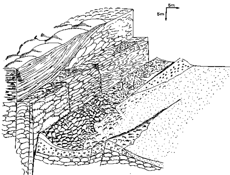
Générations de talus d'éboulis. (croquis) Ils sont séparés du mur de faille par une fissure ouverte au sommet, les laves fluides à surface lobée fossilisent les coussins anciens.
