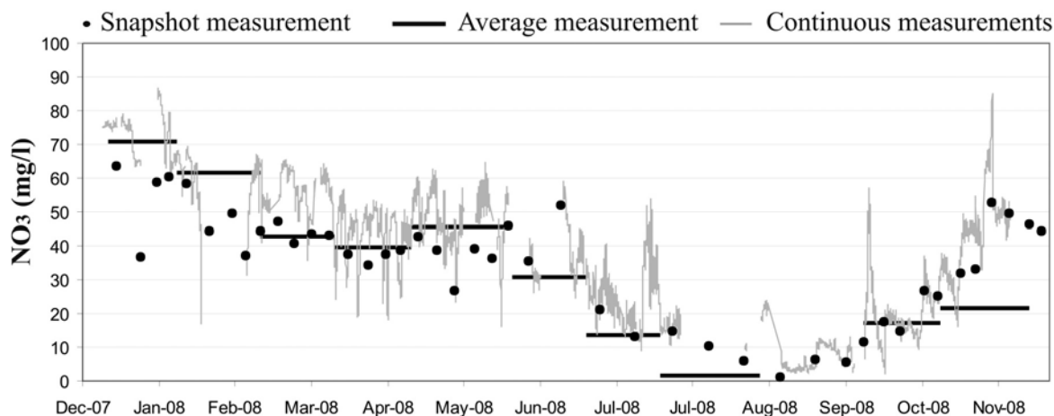
Figure 4.2. Comparaison de trois types de mesures des concentrations de \text{NO}_3^- , ponctuel, moyenné (SC Sampler) et continu. Source : Rozemeijer et al., 2010.
