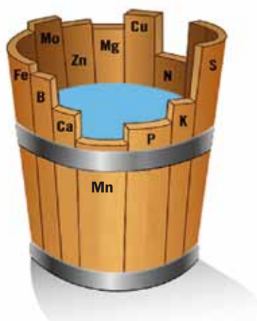
Figure 2.2. Vue schématique de la loi de Liebig du minimum (d'après Liebig vers 1850). Dans ce cas, c'est le manganèse (Mn) qui est le facteur limitant.
