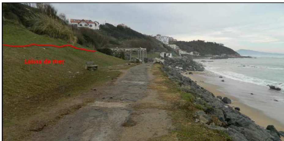
Figure 70 : Jet de rive identifiable par la laisse de mer sur le versant surplombant le sentier du littoral de Parlementia (Bidart, 09/01/2014, BRGM).
