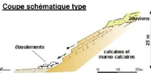
Figure 22 : Gauche : glissement banc sur banc au Nord de la Plage du Centre à Bidart ; Droite : coupe schématique type de ce tronçon littoral (Nédellec et al., 2005).
