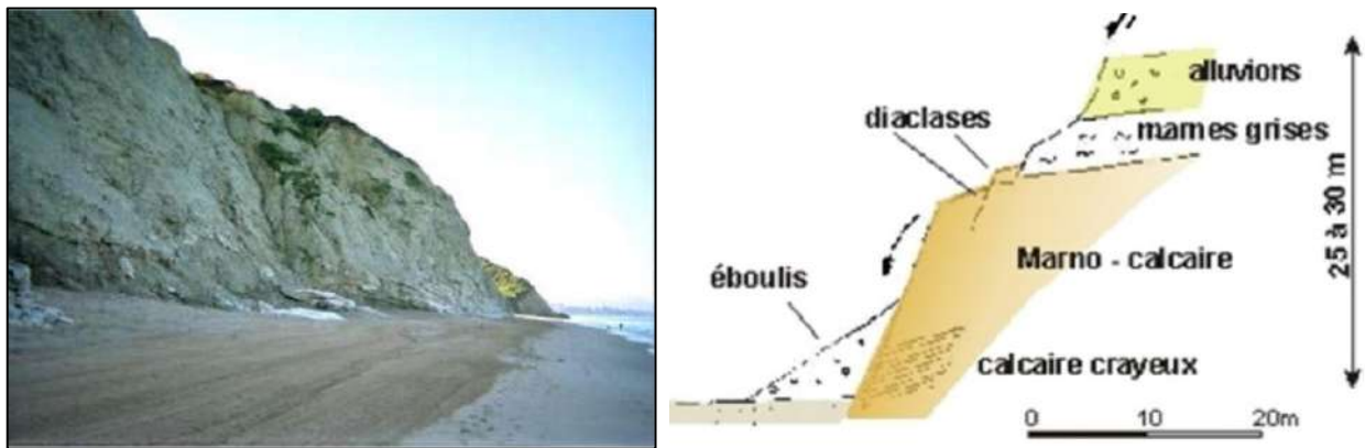
Figure 34 : Coupe schématisée de la falaise au droit du plateau de Bellevue sur la plage de Pavillon Royal (Aubié, 2008).
