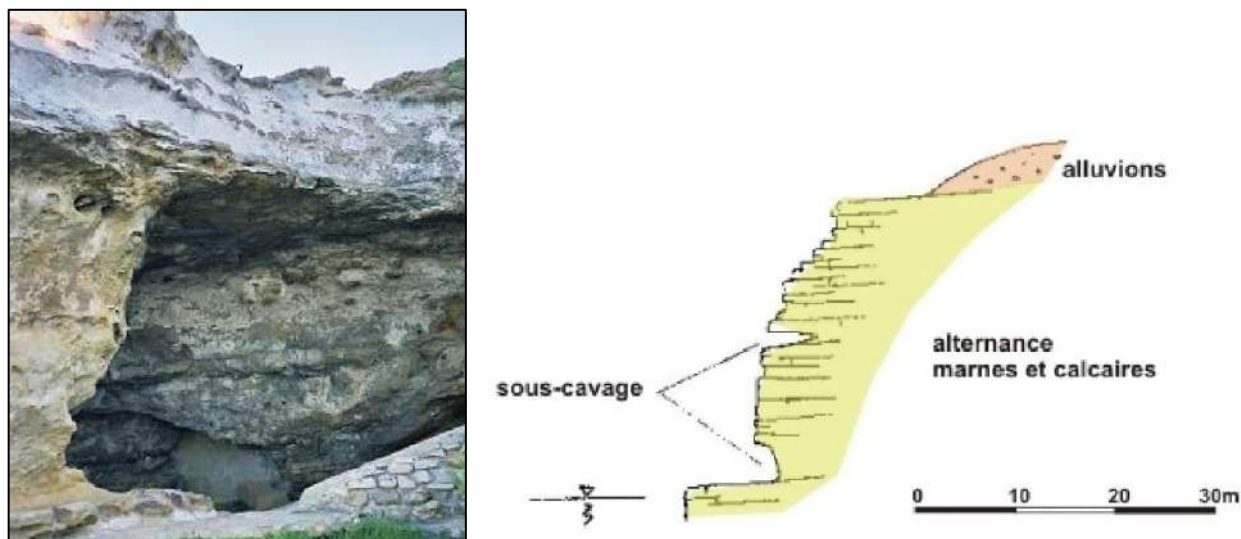
Figure 20 : Gauche : sous-cavage des bancs calcaires à la base de la Pointe Saint-Martin sur la commune de Biarritz (© Observatoire de la Côte Aquitaine) ; Droite : coupe schématique type de ce tronçon littoral (Nédellec et al., 2005).
