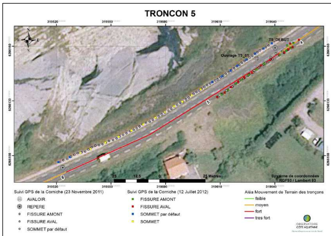
Illustration 6 : Levé DGPS 2011 et 2012 des fissures sur chaussée - tronçon 5
