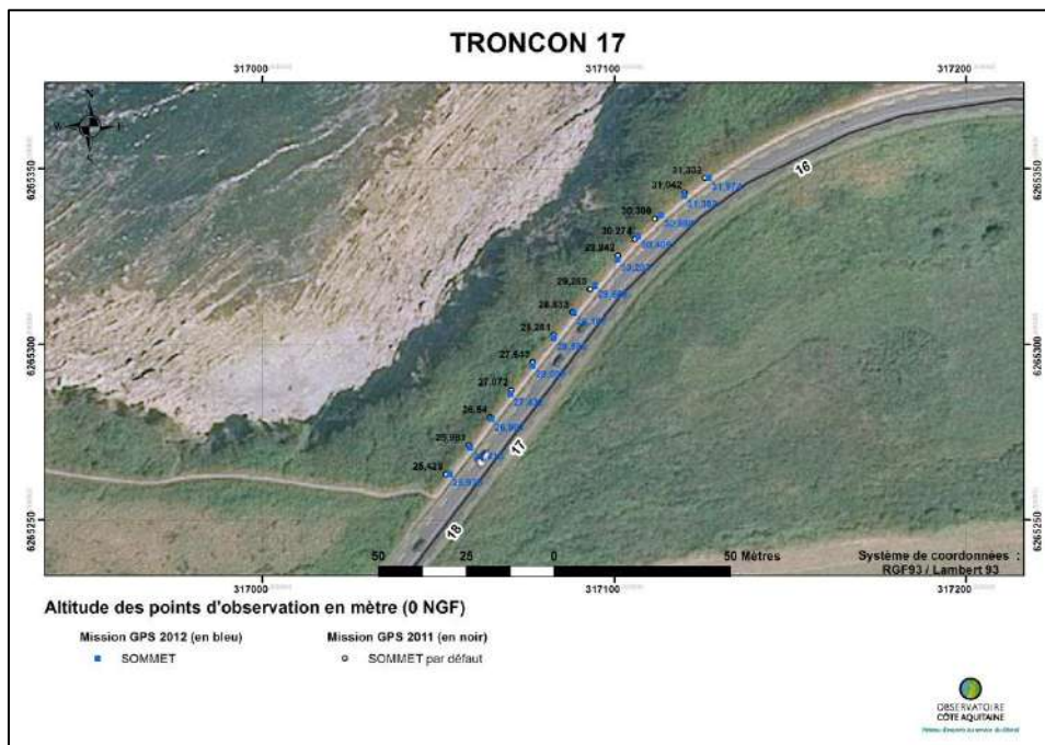
Illustration 16 : Résultats des levés DGPS 2011 et 2012 en planimétrie - tronçon 17
