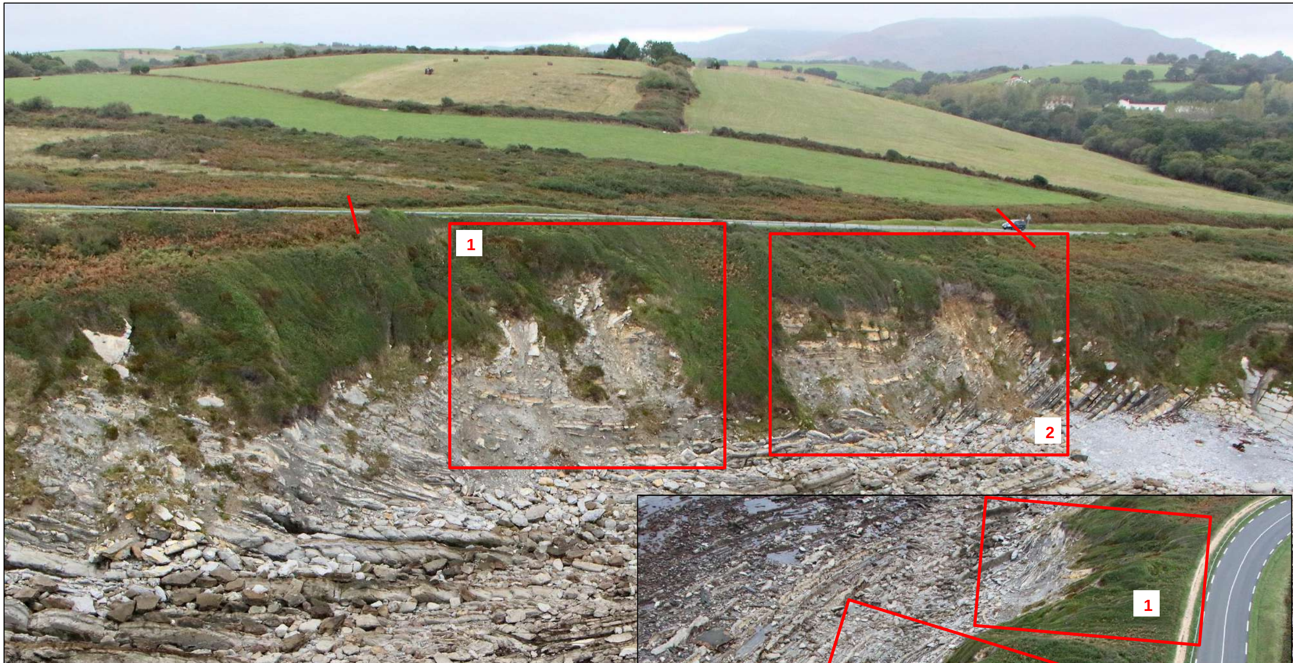
Illustration 54 : Vues générales du tronçon 17 - campagne 18/10/12
