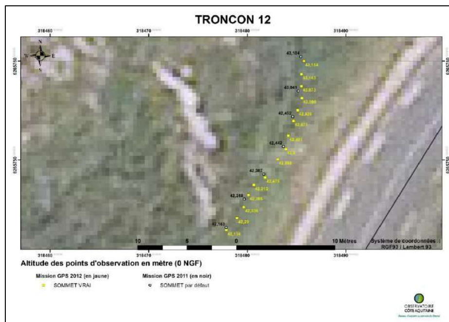
Illustration 12 : Résultats altimétriques des levés DGPS 2011 et 2012 - tronçon 12
