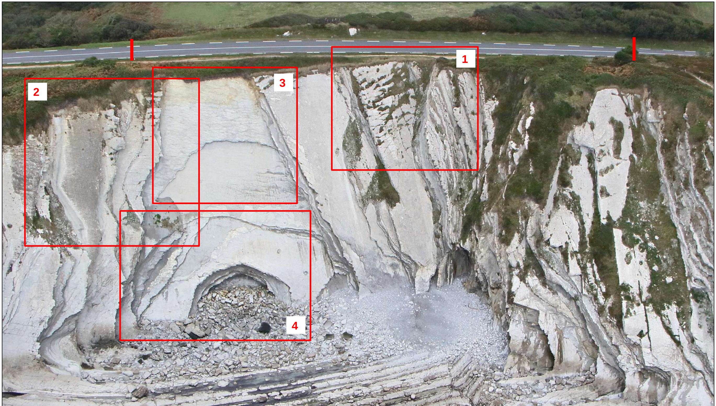
Illustration 36 : Vue générale du tronçon 9 - campagne 18/10/12
