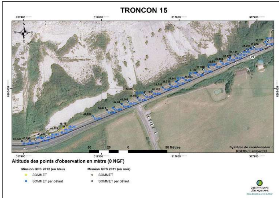
Illustration 14 : Résultats des levés DGPS 2011 et 2012 en planimétrie - tronçon 15
