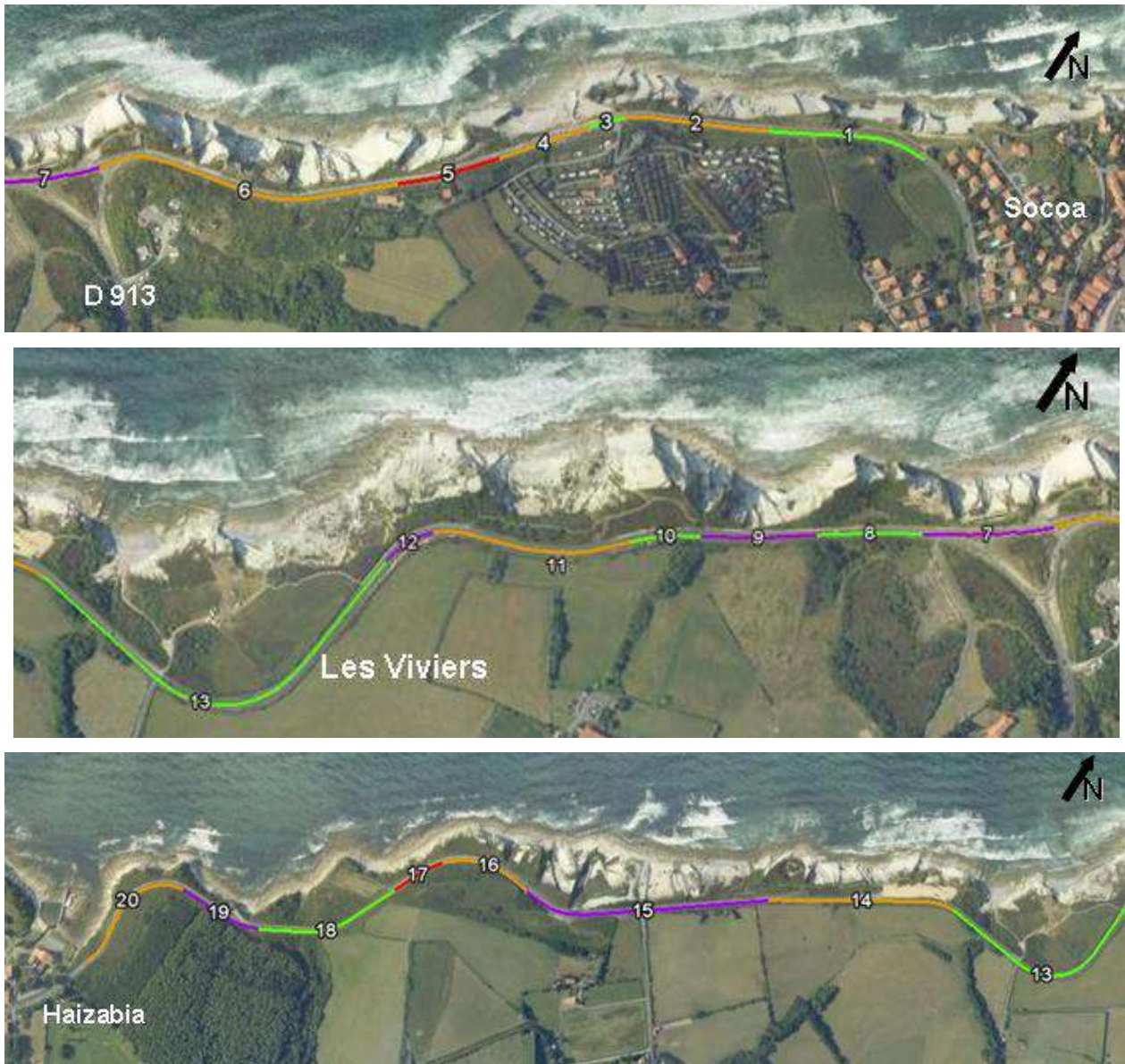
Illustration 3 : Identification des différents tronçons de la route de la Corniche et qualification de l'aléa mouvements de terrain (vert = aléa faible, orange = aléa moyen, rouge = aléa fort, violet = aléa très fort)
