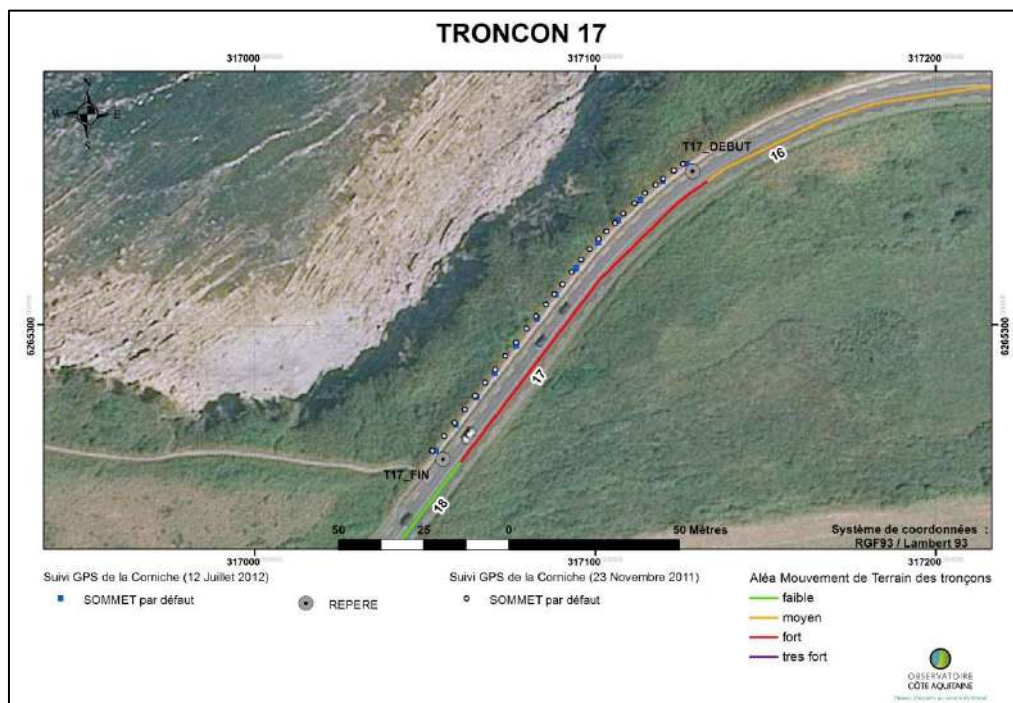
Illustration 15 : Levé DGPS 2011 et 2012 - tronçon 17
