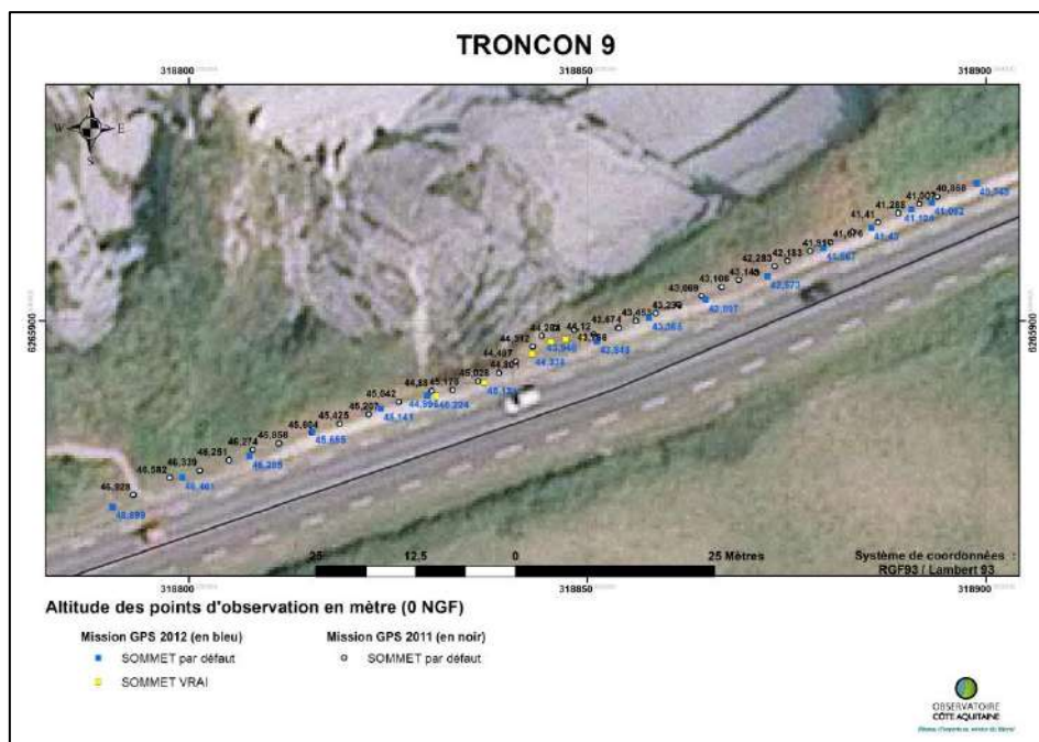
Illustration 10 : Résultats altimétriques des levés DGPS 2011 et 2012 - tronçon 9
