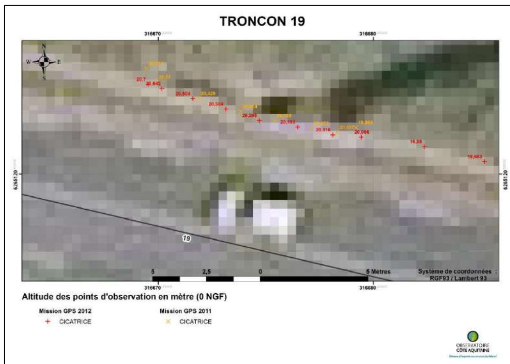
Illustration 19 : Résultats des levés DGPS 2011 et 2012 en planimétrie – cicatrice de glissement sur le tronçon 19
