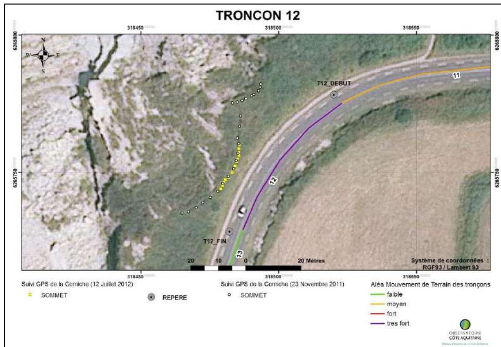
Illustration 11 : Levé DGPS 2011 et 2012 - tronçon 12
