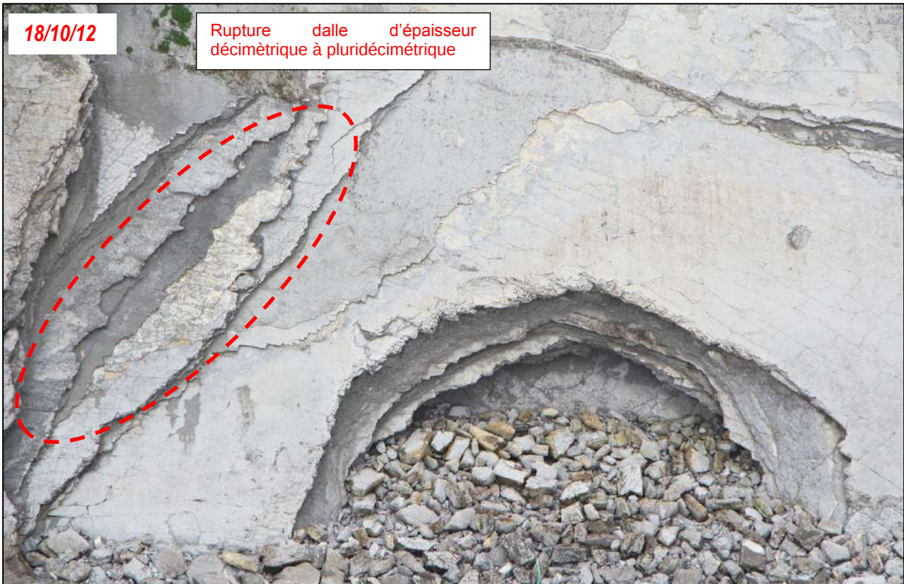
Illustration 40 : Vues de détail zone 4 - tronçon 9
