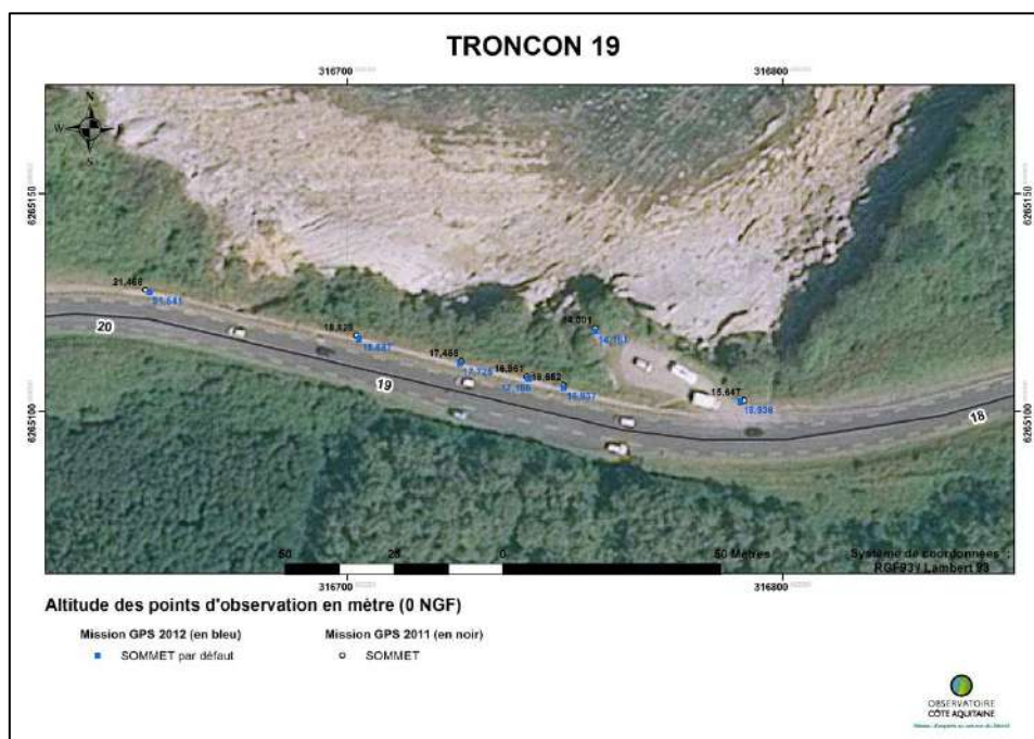
Illustration 18 : Résultats des levés DGPS 2011 et 2012 en planimétrie - tronçon 19
