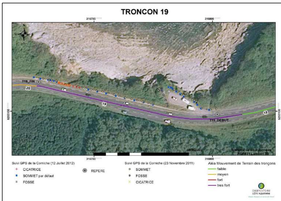
Illustration 17 : Levé DGPS 2011 et 2012 - tronçon 19
