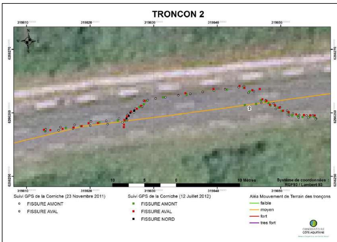
Illustration 5 : Levé DGPS 2011 et 2012 des fissures sur chaussée - tronçon 2
