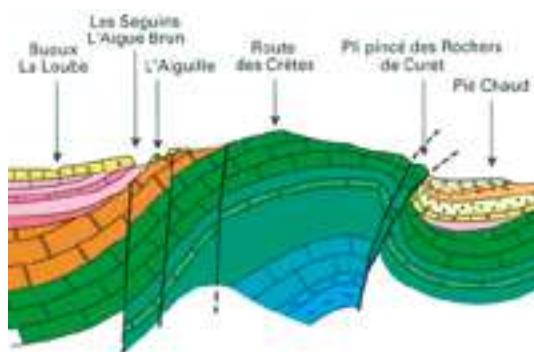
Coupe géologique du Luberon soulignant l'aspect conforme de son relief (d'après Michel Liouville)
