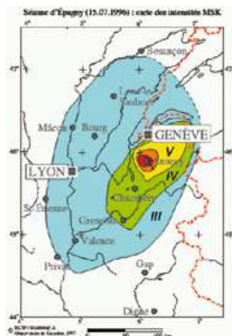
Carte isoséiste du séisme d'Annecy-Epagny du 15 juillet 1996
