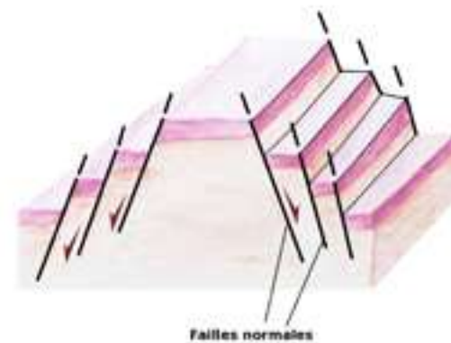
Schéma simplifié d'un horst
