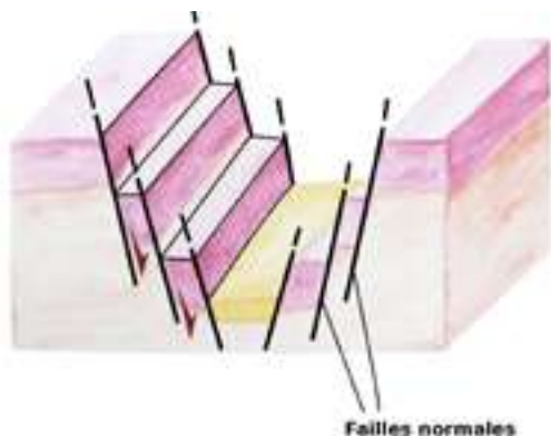
Schéma d'un fossé d'effondrement
