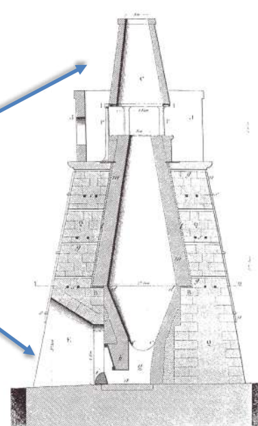
Coupe du haut fourneau de Banca.
