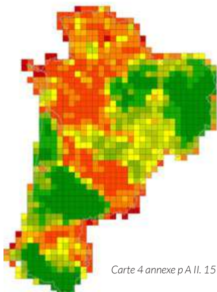
Fragmentation des espaces naturels et semi naturels
