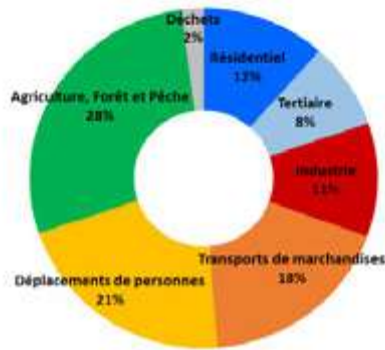
Émissions de GES par secteur en 2017
