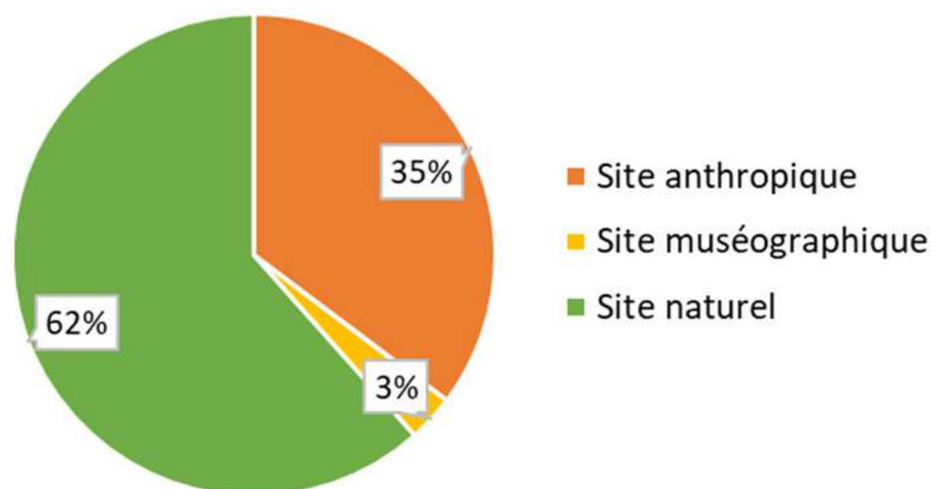
Type des sites géologiques en Nouvelle-Aquitaine (source : INPG, DREAL NA, janvier 2021)
