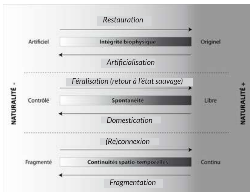
Gradients des trois composantes de la naturalité
