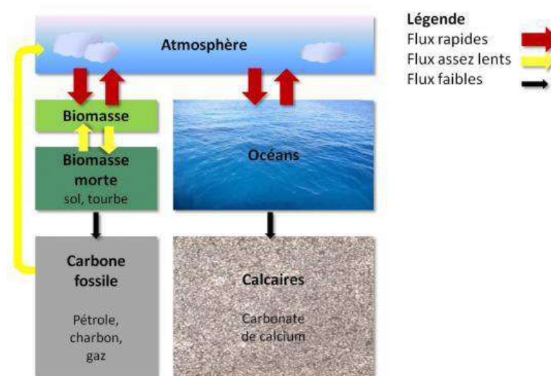
Figure 18 : Cycle du Carbone (extrait de https://www.les-crises.fr/climat-4-cycle-carbone/ )
