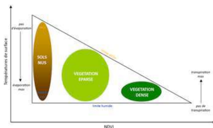
Figure 57 : Relation simplifiée entre la température de surface et l'indice de végétation (d'après Lambin et Erlich, 1996)
