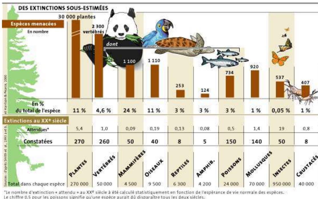
Figure 51 : Évaluation de l'extinction actuelle, pour les différents groupes animaux
