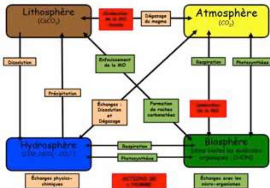
Figure 34 : Schéma simplifié du cycle du carbone
