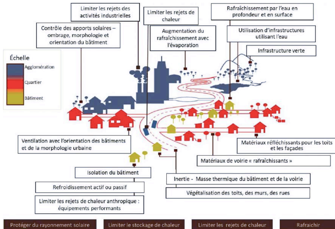
Figure 56 : Solutions pour diminuer l'intensité des îlots de chaleur (d'après Shaw et al. , 2007 et Colombert, 2016)
