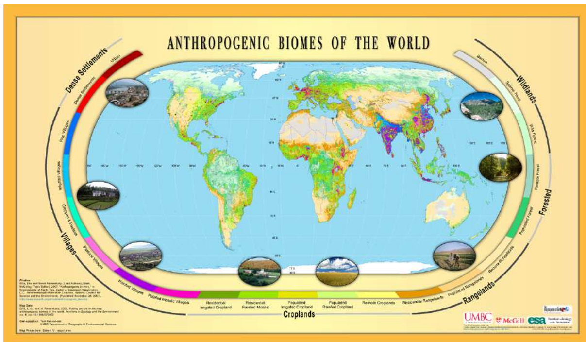
Figure 8 : Répartition des biomes anthropogéniques dans le Monde
