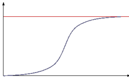
Figure 36 : Relation entre la capacité du milieu et les effectifs
