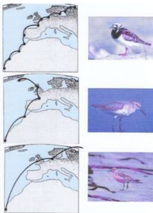
Figure 61 : Illustration des trois stratégies de migration (de haut en bas, hop, step, jump), repris de Theunis Piersma
