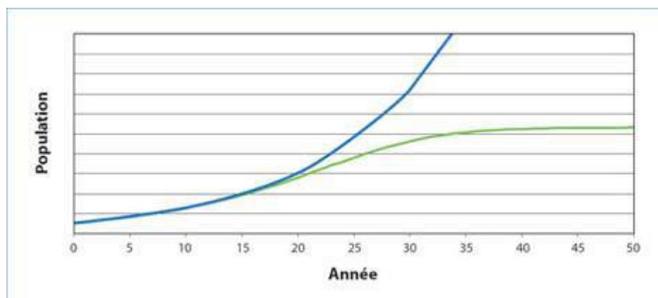
Figure 37 : Densité indépendance et densité dépendance
