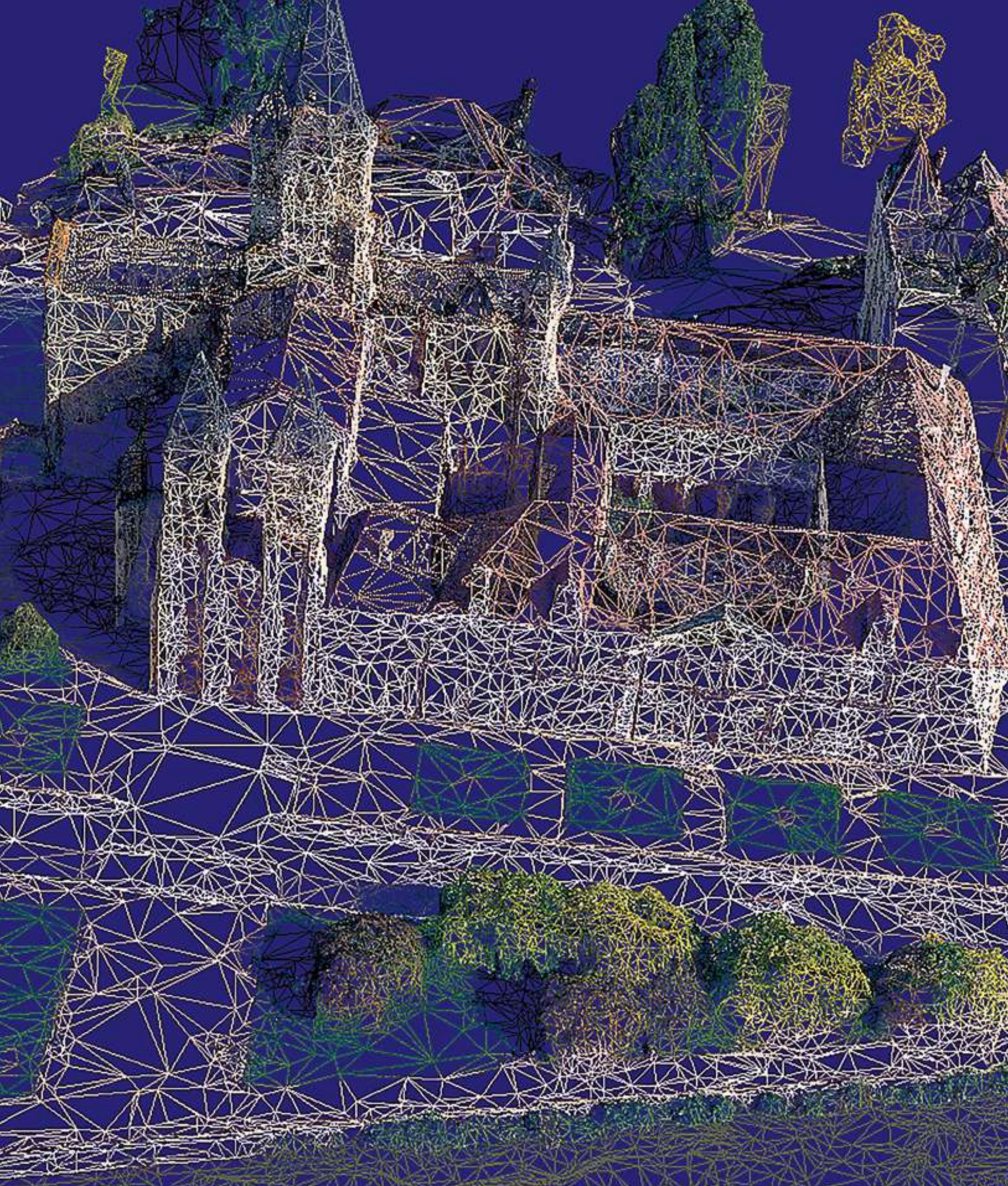
MODÉLISATION DU SOCLE 3D POUR LE FUTUR JUMEAU NUMÉRIQUE LIEU : PÉRIGUEUX (DORDOGNE) Date : 2023
