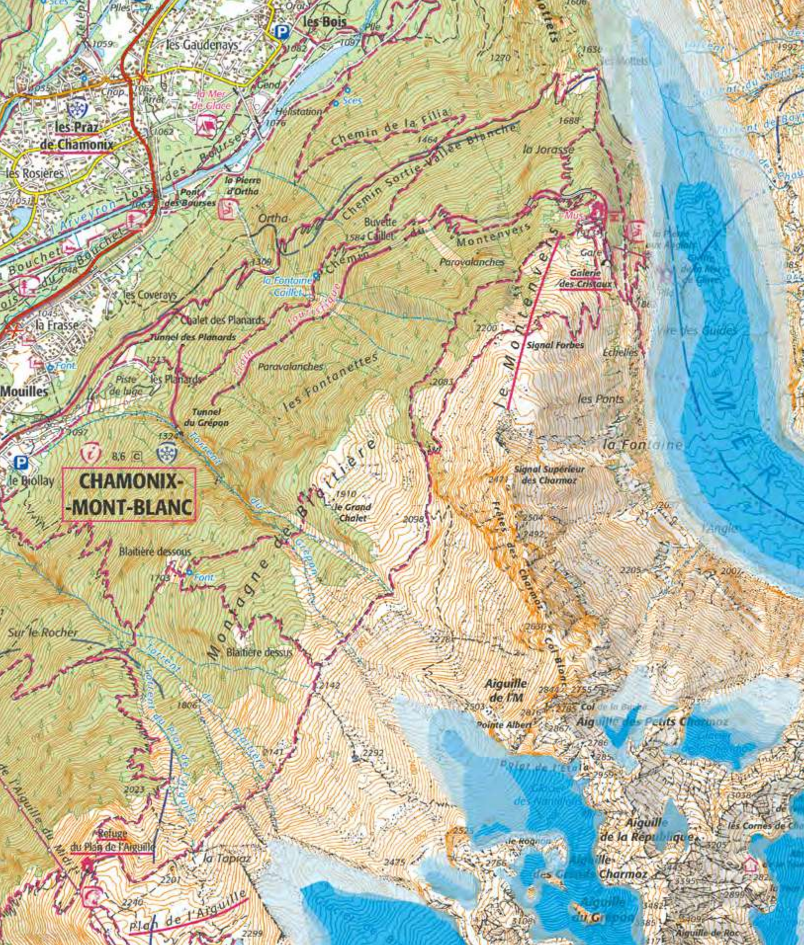
RECUL DU GLACIER DE LA MER DE GLACE LIEU : MONT-BLANC (HAUTE-SAOIE) Dates : 1937, 1980, 2011, 2023
