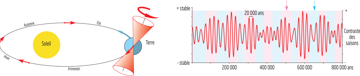
PRÉCESSION de l'axe de rotation et ROTATION de l'orbite terrestre
