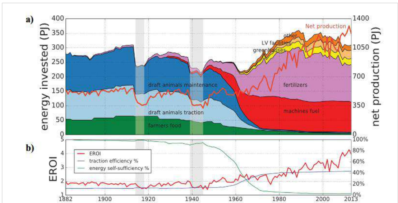
Figure 24 : a) Énergie investie par source et production nette (petajoules – PJ) et b) Retour énergétique sur énergie investie et autosuffisance énergétique
