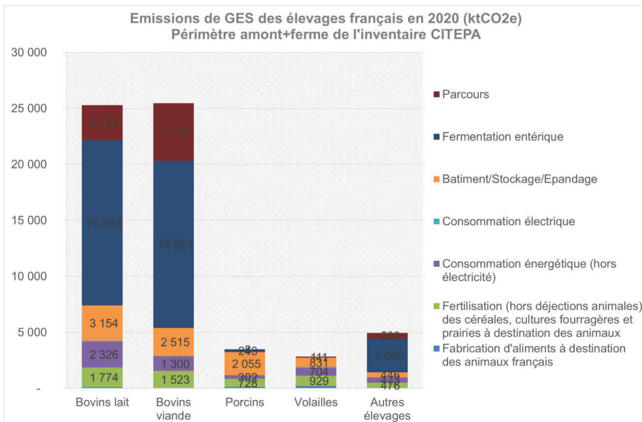
Émissions de GES des élevages français en 2020 (périmètre amont et ferme de l'inventaire CITEPA) Source CITEPA 498
