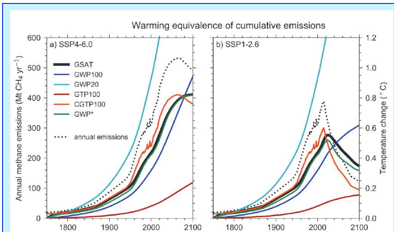
Figure 39 : comparaison des courbes d'impact passée et projetées des émissions de méthane, en référence à la modélisation GSAT en mobilisant différentes métriques, dont le PRG*, le PRG100 et le PRG20. La courbe de référence est celle en traits pleins noirs. GWP correspond à PRG.
