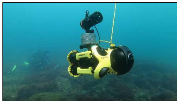
Figure 10. Drone sous-marin Chasing M2 ® avec ses accessoires et sa mise en œuvre dans l'eau © Ifremer.
