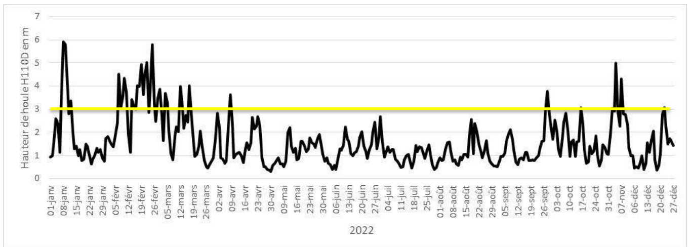
Figure 31. Épisodes de houle ; H110D = Moyenne des périodes du dixième supérieur en hauteur des vagues définies par passage au niveau moyen par valeurs décroissantes.
