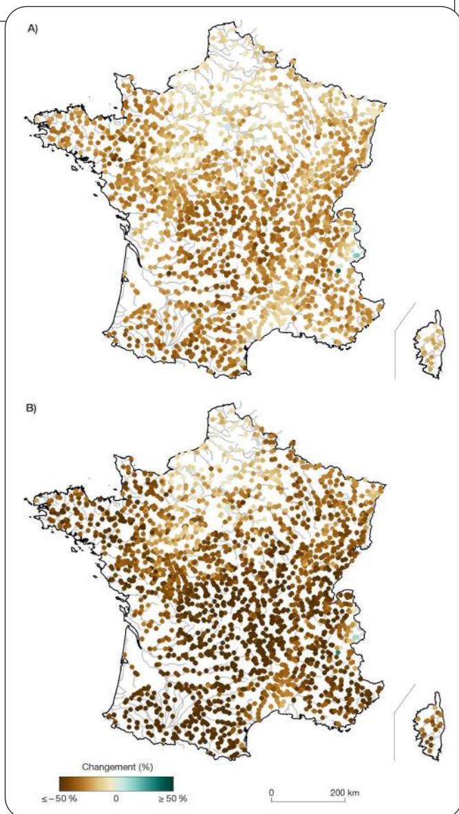
Figure 1.4. Changements projetés pour la moyenne des débits d'étiage VCM10 estival sous scénario RCP4.5 (A) et RCP8.5 (B) en fin de siècle (période de référence : 1976-2005) (estimation médiane toutes projections confondues).
