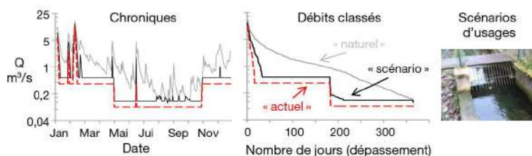
Figure 3.2. La démarche de définition des débits écologiques utilisée en France, d'après Lamouroux et al. (2018).
