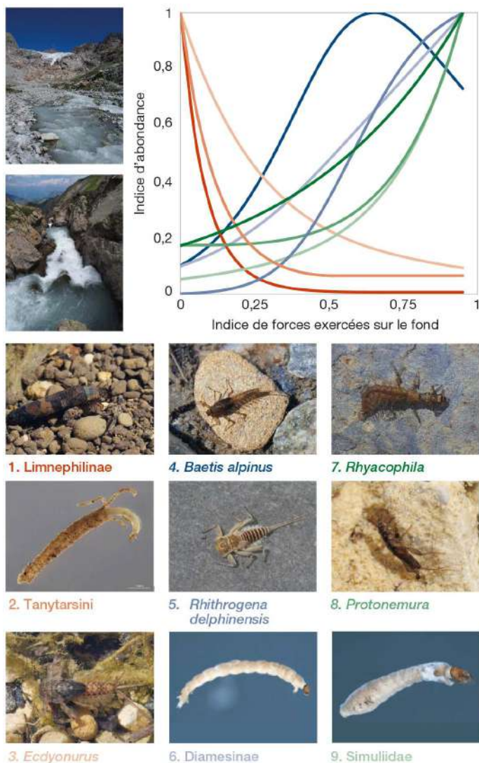
Figure 3.4. Exemples de modèles de sélection de l'habitat hydraulique par les macroinvertébrés des cours d'eau de montagne, reliant un indice d'abondance des taxa (score entre 0 et 1, 1 étant l'abondance maximale observée) à la force exercée sur le fond (score entre 0 et 1, 1 étant la force maximale observée). Photographies : © Bertrand Launay, Sophie Cauvy-Fraunié, Maxence Forcellini.
