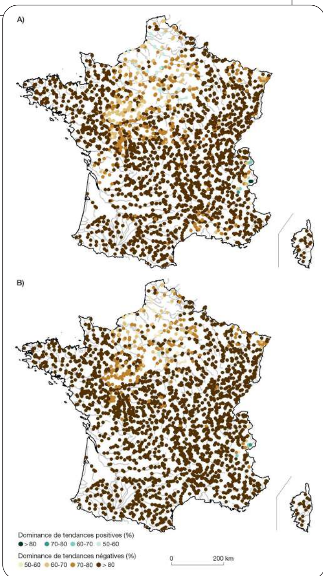
Figure 1.3. Signe majoritaire et proportion associée des tendances sur l'ensemble du xxI^e siècle pour le débit d'étiage VCN10 sous scénarios RCP4.5 (A) et RCP8.5 (B) (toutes projections confondues).
