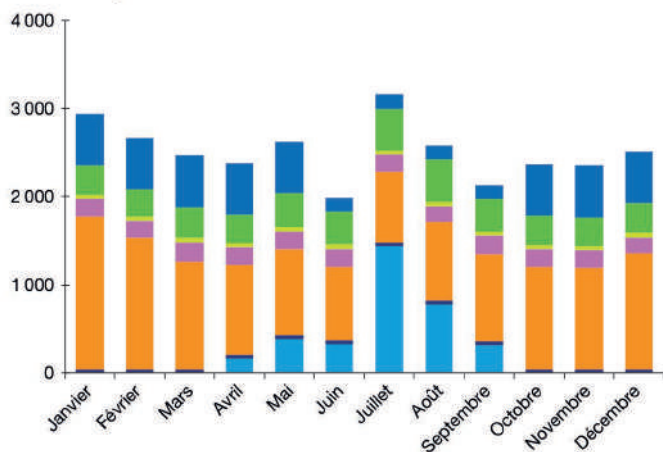
Figure 2.8. Prélèvements (A) et consommations (B) mensuelles en 2020 en France hexagonale et Corse, estimés à partir du logiciel Strateau (en millions de mètres cubes).
