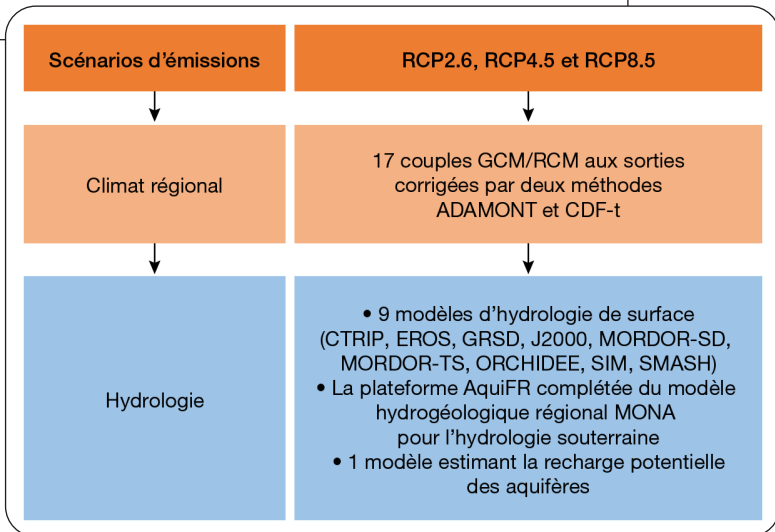
Figure 1.2. Chaîne de modélisation retenue pour le projet Explore2.
