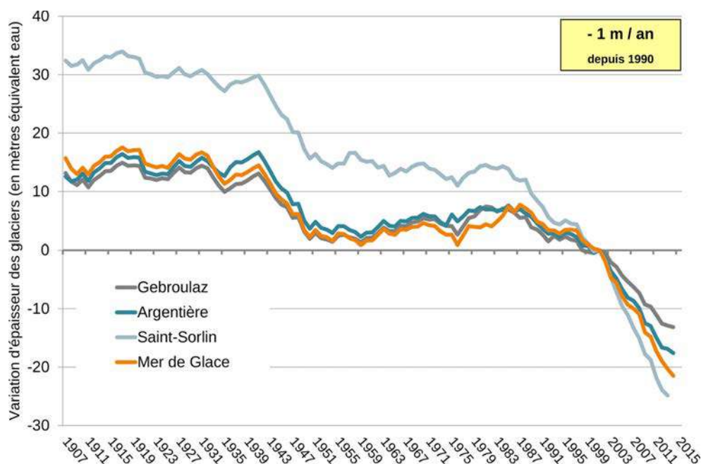
Graphique 22 : Évolution de la variation d'épaisseur des glaciers métropolitains
