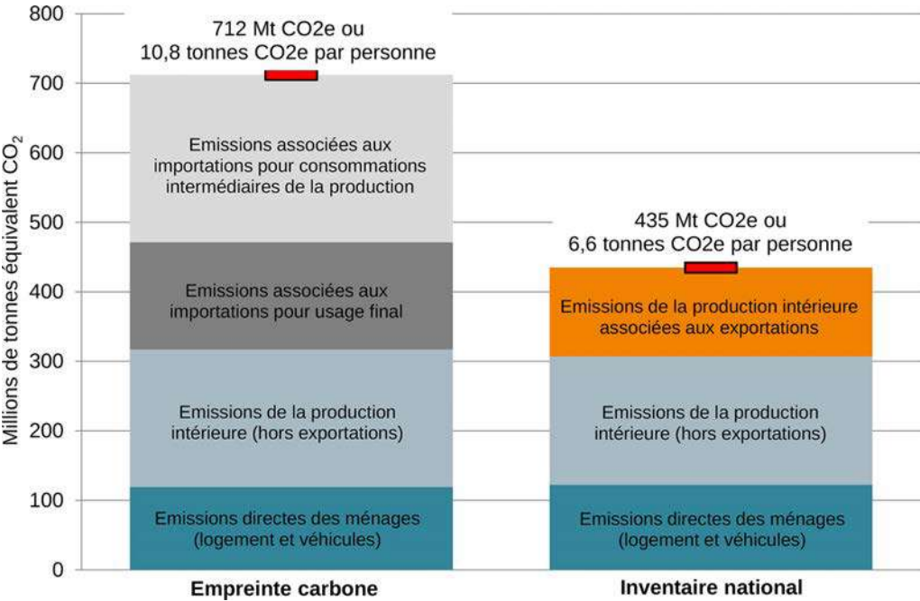
Graphique 26 : Comparaison de l'empreinte carbone et de l'inventaire national en 2014
