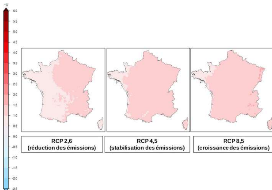
Image 2 : Écarts de températures à l'horizon 2021-2050 par rapport à la période 1976-2005 – Moyenne annuelle selon différents scénarios d'émissions de GES
