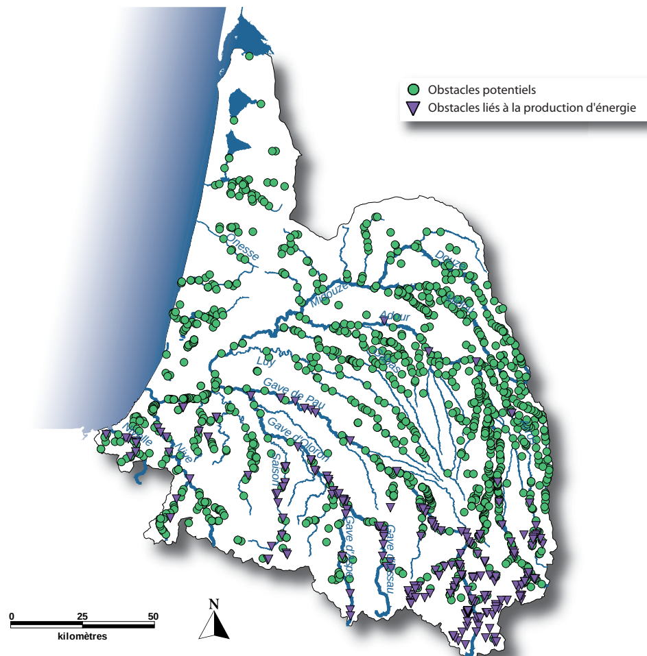
Ouvrages recensés sur les cours d'eau du territoire du PLAGEPOMI Adour et cours d'eau côtiers. Identification des ouvrages hydroélectriques. (Sources : Réseau des Obstacles à l'Écoulement ONEMA).
